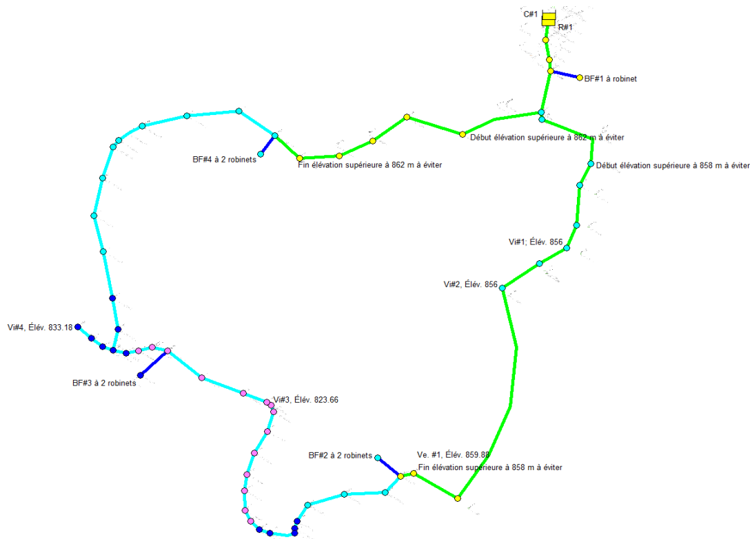
Vue d'ensemble du réseau de distribution projeté pour l'alimentation de Miguel
